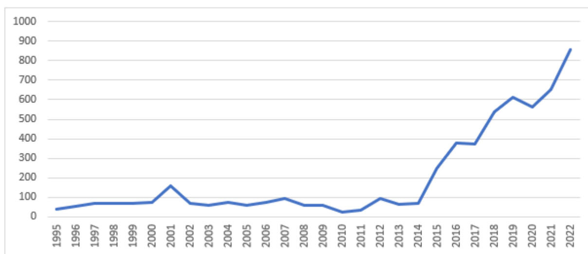
Figur 1: Årsimport (i ton) av lustgas till Sverige.
